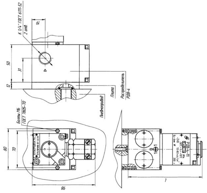
Габаритные и установочные размеры распределителей РДВ-4-11, РДВ-4-13, РДВ-4-14, РДВ-4-15, РДВ-4-16, РДВ-4-17 со стыковой поверхностью NAMUR
